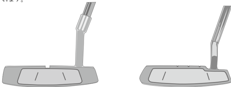
図34 ヘッドの上部あるいはクラウンにフェースまで及んでいる機構があるパターの例。こうした機構は0.25インチ（6.35ミリメートル）を超える深さがない限りは認められます。
